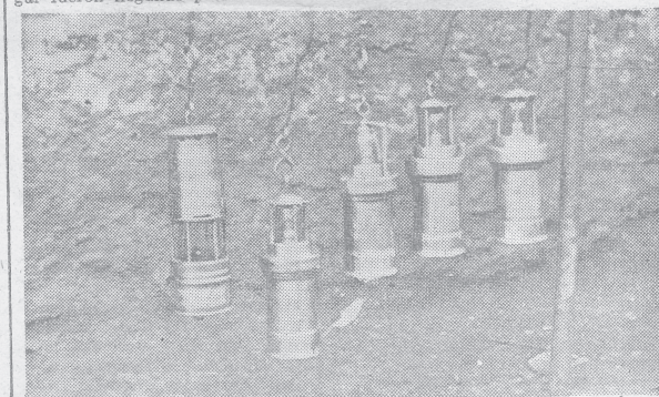
Estas son las lámparas de seguridad utilizadas en la mina de Ocejón.
